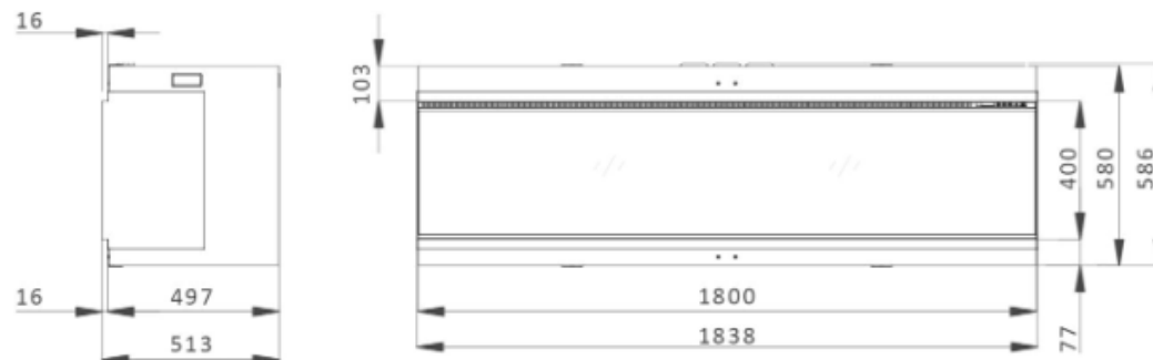
Dimensions
